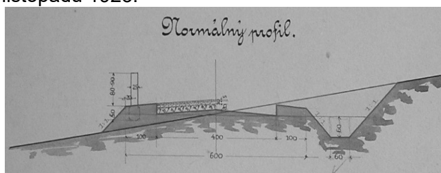
Obr. č. 8. Na obrázku je jeden z profilů silnice, kterou obec vlastními silami postavila
